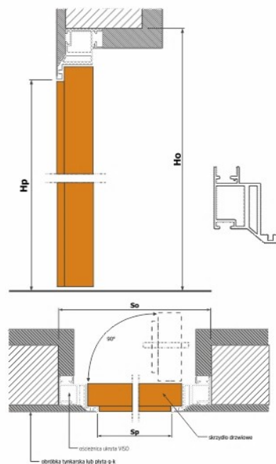
VISIO 40 - WEWNĘTRZNE
